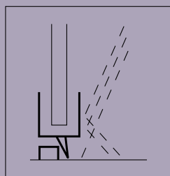
Gulvprofilsett med drypplst og gulvlist til dusjløsninger med svingdører. (Kjøpes separat).
